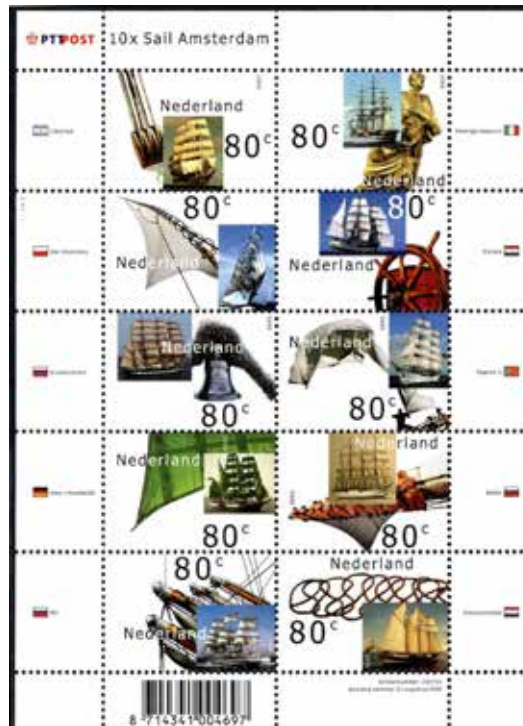
k 128
